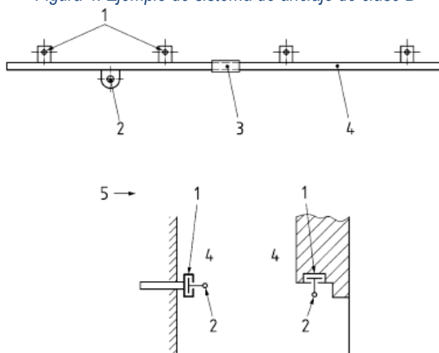
Figura 4. Ejemplo de sistema de anclaje de clase D
